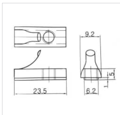
SPRING NUT(M6)
